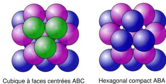
Cubique à faces centrées ABC
